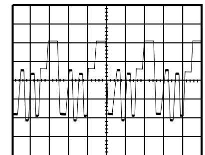
WF13 1DIV: 20V 20μsec Q1532 Collector
